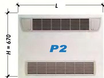
Dimensioni nicchia (per installazione senza FTI) - Nike dimensions (for installation without FTI) ( Ln ) x ( Hn = 620 ) x ( Sn = 220 )
