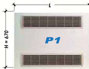
Dimensioni nicchia (per installazione senza FTI) - Nike dimensions (for installation without FTI) ( Ln ) x ( Hn = 620 ) x ( Sn = 220 )
